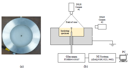
Rys. 3. (a) Próbkę z polietylenu otoczona uziemionym pierścieniem, (b) układ eksperymentalny inicjujący wyładowania powierzchniowe na badanej próbce, [3]
