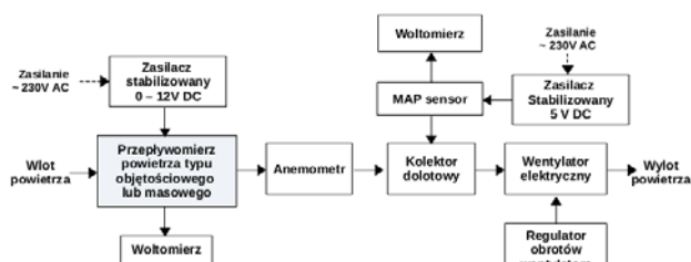
Rys. 4. Schemat blokowy stanowiska do badania przepływomierzy powietrza
