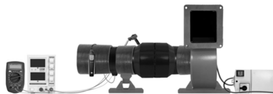
Rys. 6. Stanowisko badawcze dla przepływomierza typu MAP
