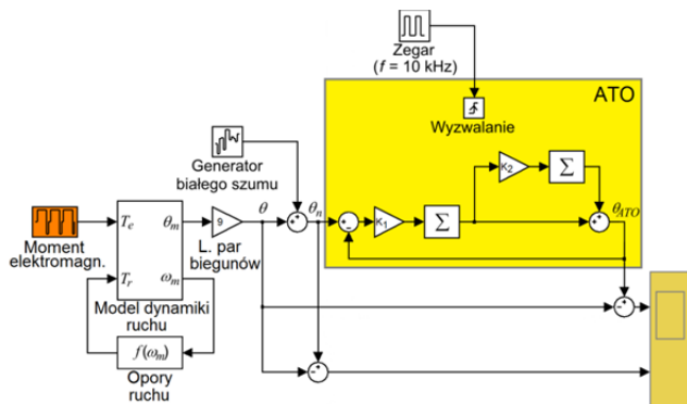
Rys.4. Schemat modelu symulacyjnego układu napędowego z zaimplementowanym obserwatorem ATO
