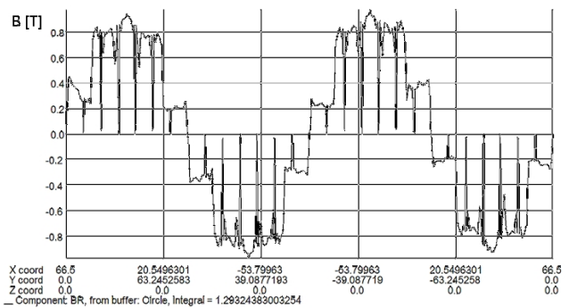
Rys. 7. Symulacja polowa pokazująca rozkład indukcji magnetycznej w szczelinie powietrznej silnika.
