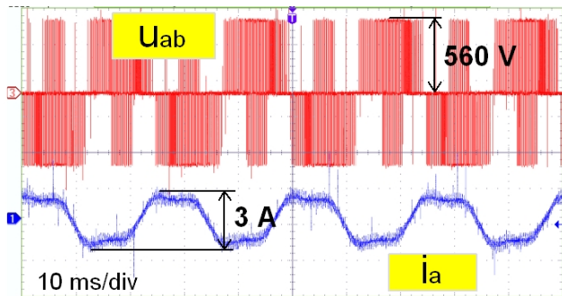
Rys.8. Przykładowe przebiegi napięcia międzyfazowego falownika oraz prądu stojana pięcioletowego silnika indukcyjnego przy wymuszaniu częstotliwości napięcia odpowiednio: 40 Hz w pierwszym układzie oraz 120 Hz w drugim układzie.
