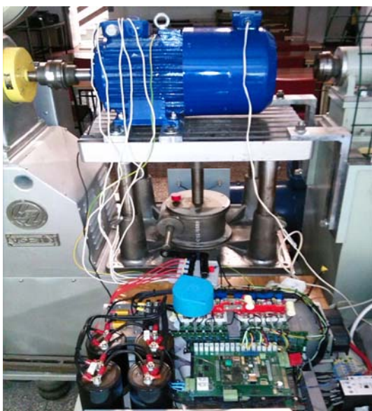
Rys.10. Widok stanowiska laboratoryjnego z badanym pięcioletowym silnikiem indukcyjnym o mocy 5,5 kW zasilanym z pięcioletowego falownika napięcia z proponowanym sterowaniem multiskalarnym.
